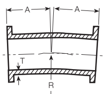
A-508 5½° Bend
