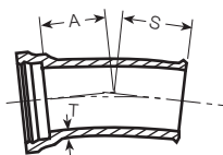
A-207 Bell & Spigot 11 1/4° Bend
