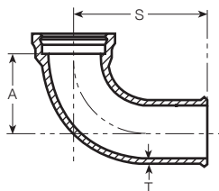
A-201 Bell & Spigot 90° Bend
