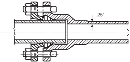
A-702 2"
