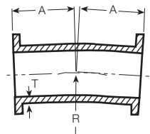
A-508 5%° Bend
