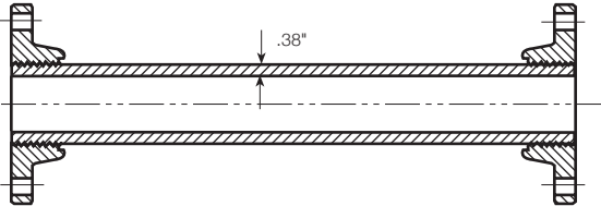
A-706 2"
