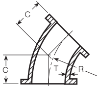
A-502 45° Bend
